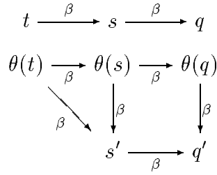
Fig. 4. Lemma 43
