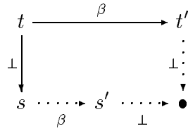
Fig. 5. Lemma 45
