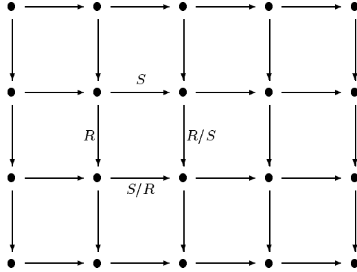
Fig. 6. A tiling diagram
