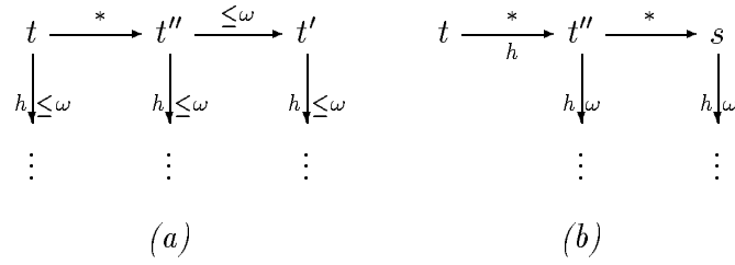
Fig. 8. Lemma 54
