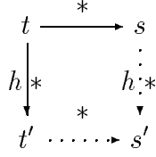
Fig. 7. Lemma 53
